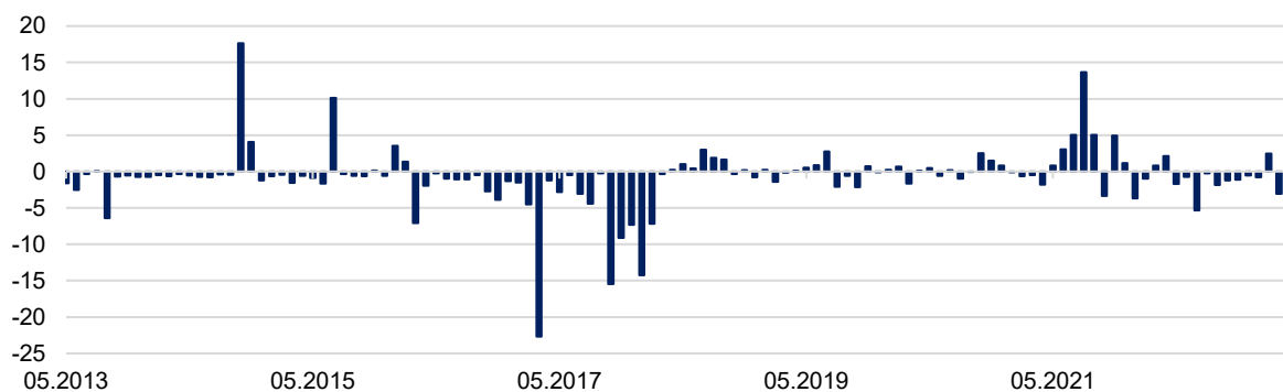
Abb. 1 | Monatliche Netto-Mittelflüsse
